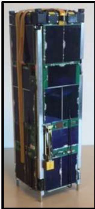
URSA MAIOR 3U CubeSat
